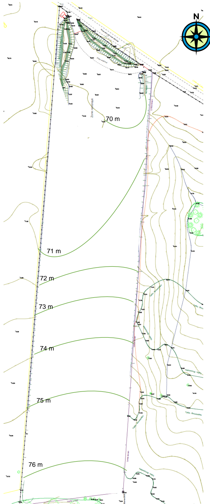
Figure 38 : Plan de remise en état agricole au 1/2000° (côtes NGF)
